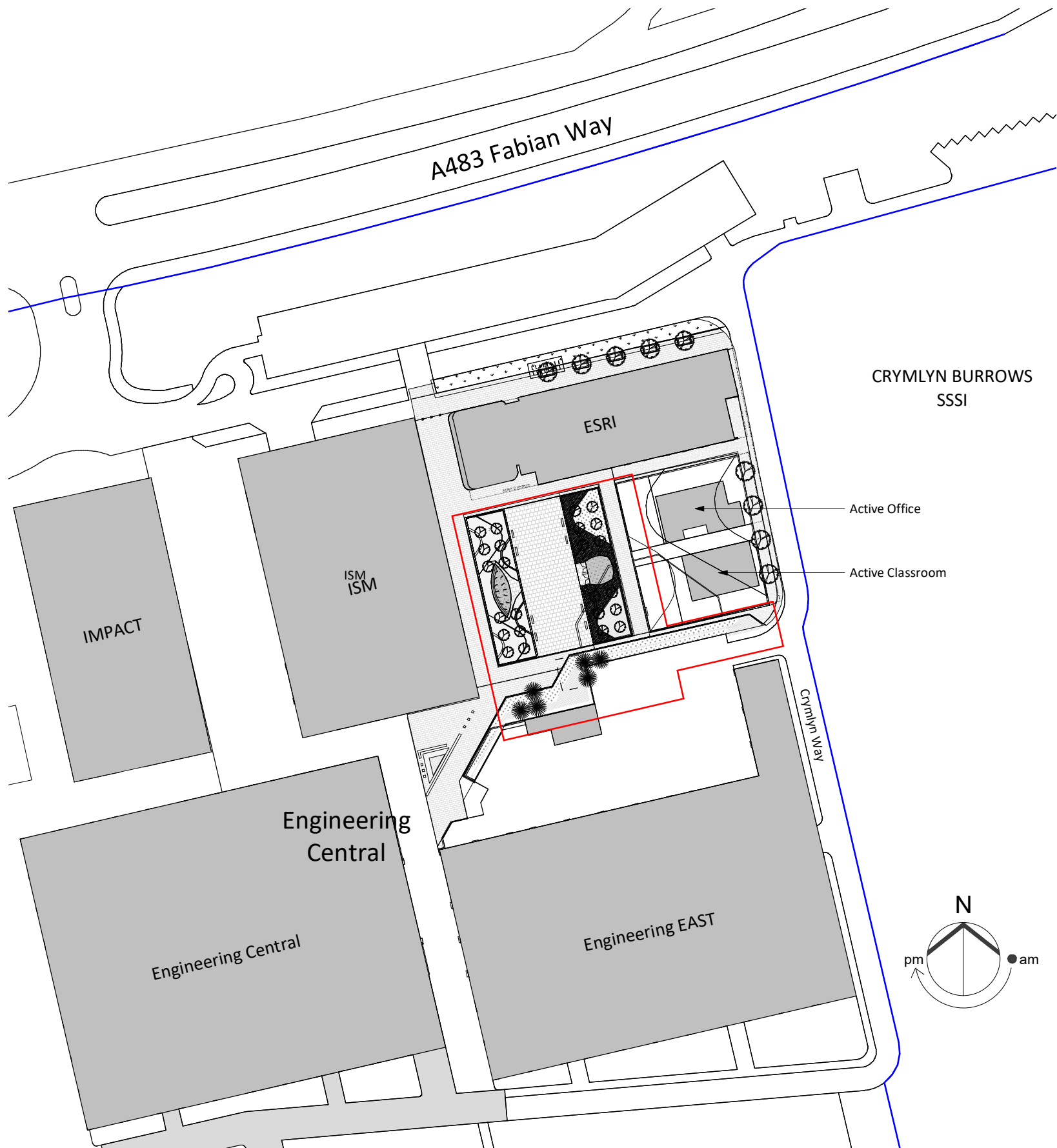
SITE PLANNING 1 : 1250
